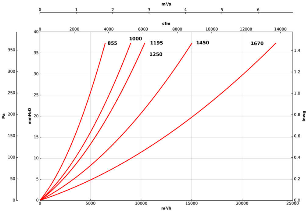
Módulos filtrantes: / Filter modules: / Filtermodule: / Modules filtrants : TPCO F7+F9
