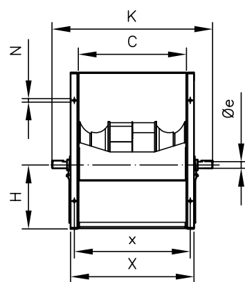
Abmessungen mm
